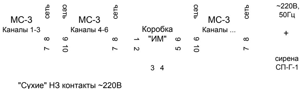
Рис. 8 - Схема соединений коробки "ИМ" для отключения исполнительного механизма при срабатывании только от каналов 1 ... 6.
